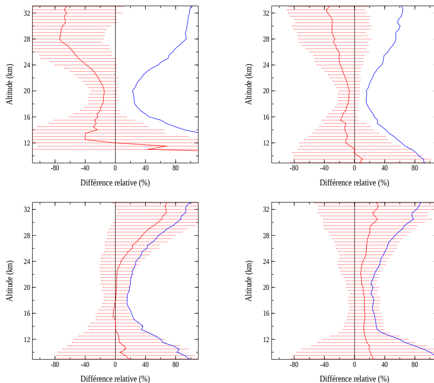
FIG. 4.51 – Identique à la figure 4.50 mais pour les coefficients d’extinction des aérosols. En haut à gauche : 384.2 nm pour SAGE III et 386 nm pour SAGE II. En haut à droite : 448.5 nm pour SAGE III et 452 nm pour SAGE II. En bas à gauche : 520.3 nm pour SAGE III et 525 nm pour SAGE II. En bas à droite : 1022.1 nm pour SAGE III et 1020 nm pour SAGE II.
