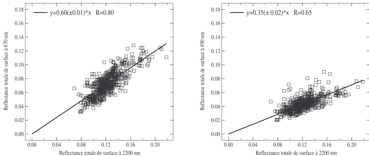
Figure V-21 : Réflectances de surfaces à 670 nm, obtenues pour le vol du 18/02/04, en fonction de la réflectance de surface à 2200 nm.
