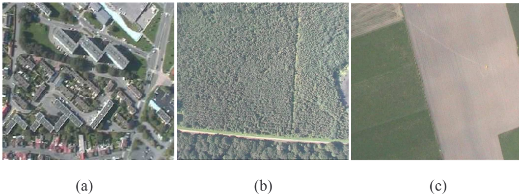
Figure V-5 : Images obtenues à l'aide de la caméra numérique pour plusieurs types de surfaces survolées (le 06/09/04).
