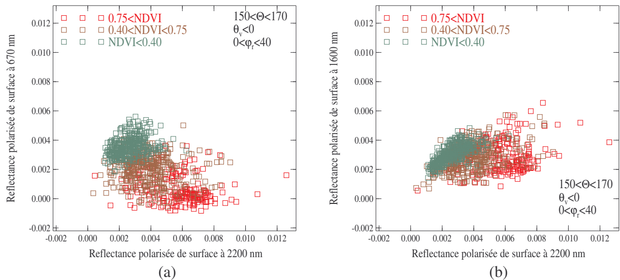
Figure V-8 : Réflectances polarisées de la surface à 670 nm (a) et 1600 nm (b) en fonction de celle à 2200 nm, obtenues en diffusion arrière ( \theta_v < 0^\circ ) et pour les trois types de surfaces survolés le 06/09/04.
